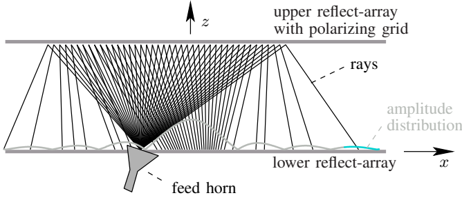
Fig. 8. Rays in the x - z -plane.
